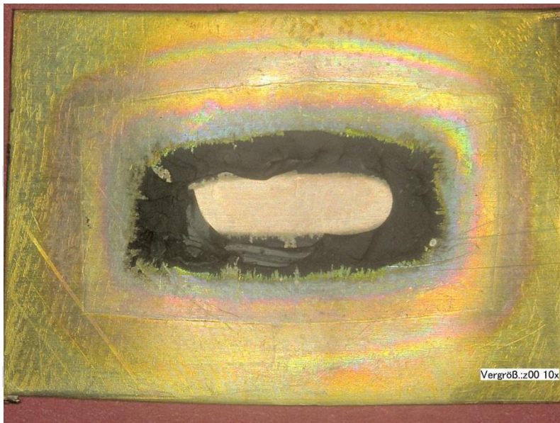
Abb. 9: Überreste einer großflächigen Verklebung eines Probekörpers auf einer Kupferplatte: Ein solches Elastomer gilt als anfällig für Autoxidation.
