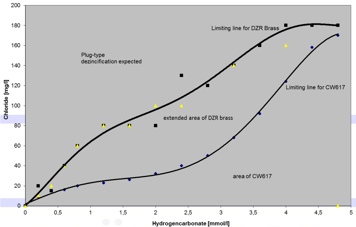
Abb. 1: Turner Diagramm mit Grenzbereichskurven zweier unterschiedlicher Messingqualitäten: Die obere Kurve steht für ein entzinkungsstabiles Messing (DZR); oberhalb dieser Kurve kommt es zur Entzinkung auch dieses stabileren Werkstoffes. Die untere Kurve steht für ein Automatenmessing (CW 617N = ähnlich der inzwischen unzulässigen Bezeichnung Ms 58), unterhalb dieser Kurve kommt es bei beiden Werkstoffen zu keiner Entzinkung (Abbildung: Werkstoffberatung Dr. Peter Dierschke)
