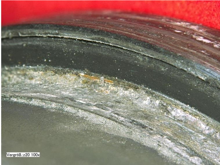
Abb. 6: EPDM- O-Ring nach Autoxidation im eingebauten Zustand, bleibend verformt und mit rußender Oberfläche
