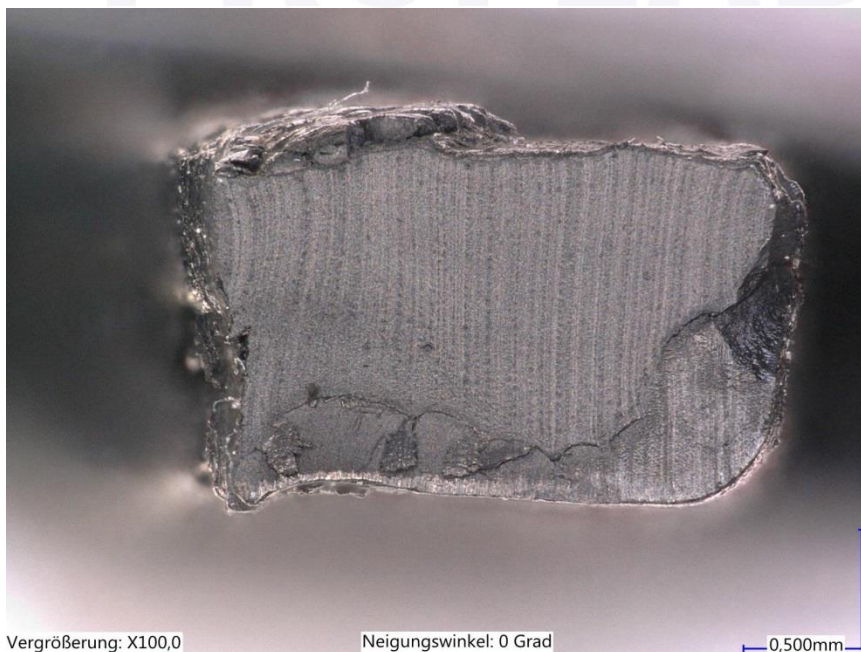
Abb. 3: Querschnitt des O-Rings aus Abb. 2, die autoxidative Schädigung fand hauptsächlich in den Randbereichen statt, der Kern ist noch nicht depolymerisiert.
