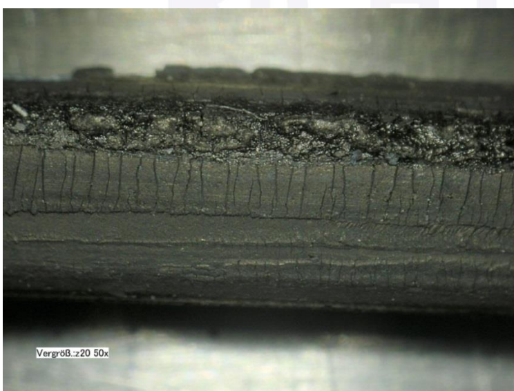
Abb. 8: Draufsicht auf ausgebauten EPDM O-Ring aus Abb. 6, gut zu erkennen sind die scheinbar angeschmolzenen Bereiche im oberen Bereich. Diese hatten Wasserkontakt, in welchem das Kautschukgift gelöst war. Die Seite mit den feinen Rissen ist die Kontaktfläche zum Gehäuse
